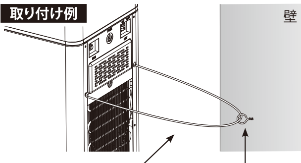
固定金具
